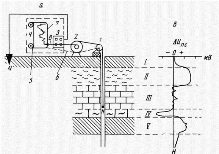
а - схема установки: 1 - блок-баланс, 2 - лебедка с коллектором, 3 - милливольтметр, 4 - регистратор, 5 - лентопротяжный механизм, соединенный гибким валиком (6) с роликом блок-баланса, 7 - диаграммная бумага, 8 - карандаш; б - диаграмма естественных потенциалов по стволу скважины: I (почва) и III (известняки) - пласты со слабой электрохимической активностью, II (суглинки) и V (глины) - пласты с положительными аномалиями ПС, IV - пласт с отрицательной аномалией ПС, характерной для проницаемых слоев
