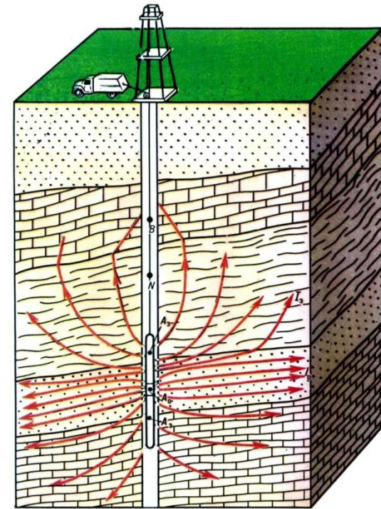
А 0 - основной токовый электрод; А э - экранированный электрод; В - обратный токовый электрод; N - обратный измерительный электрод; I 0 - токовые линии основного токового электрода; I э - токовые линии экранированного электрода.
