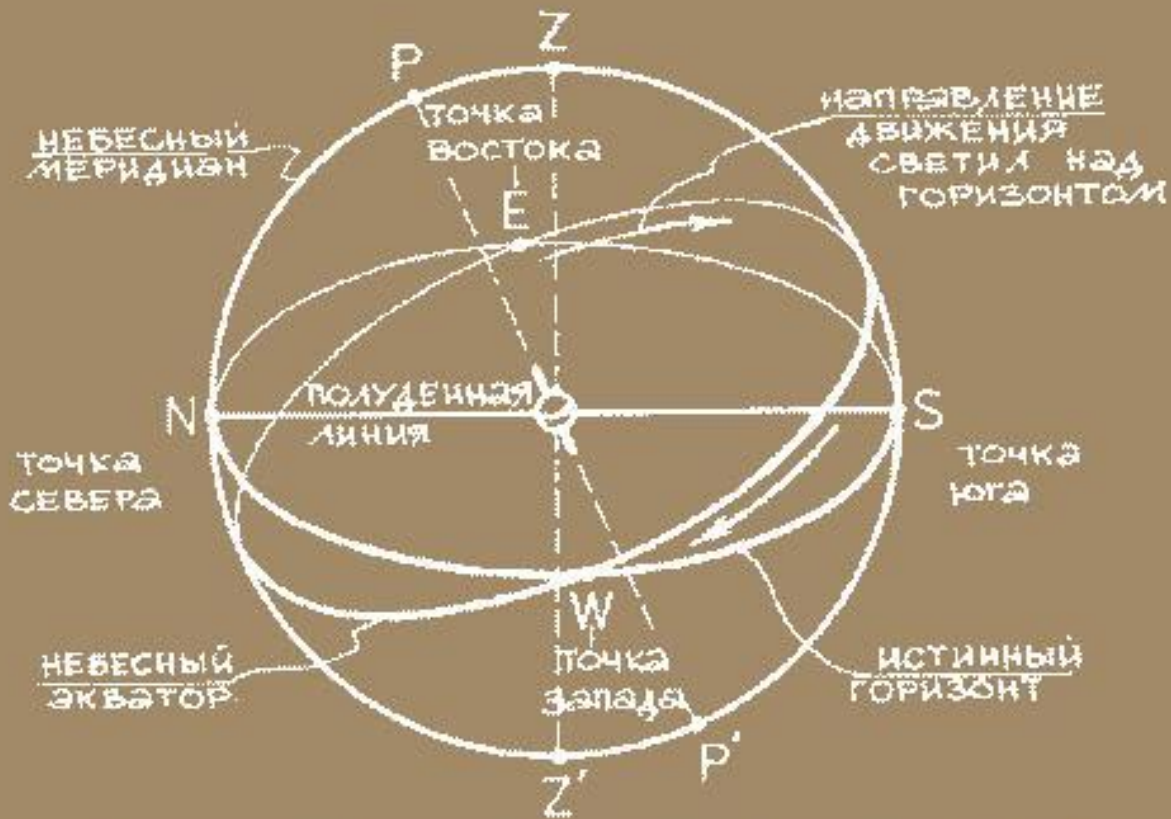
Пересечение небесного экватора и небесного меридиана с истинным горизонтом
