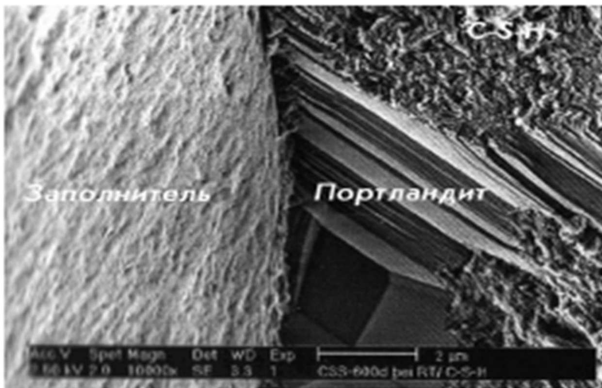
Рисунок 4 – Гель С-С-Н и сrostки кристаллов портландита в структуре затвердевшего камня. Снимок сделан с помощью СЭМ.
