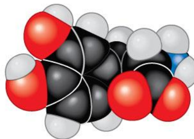
D-dopa
