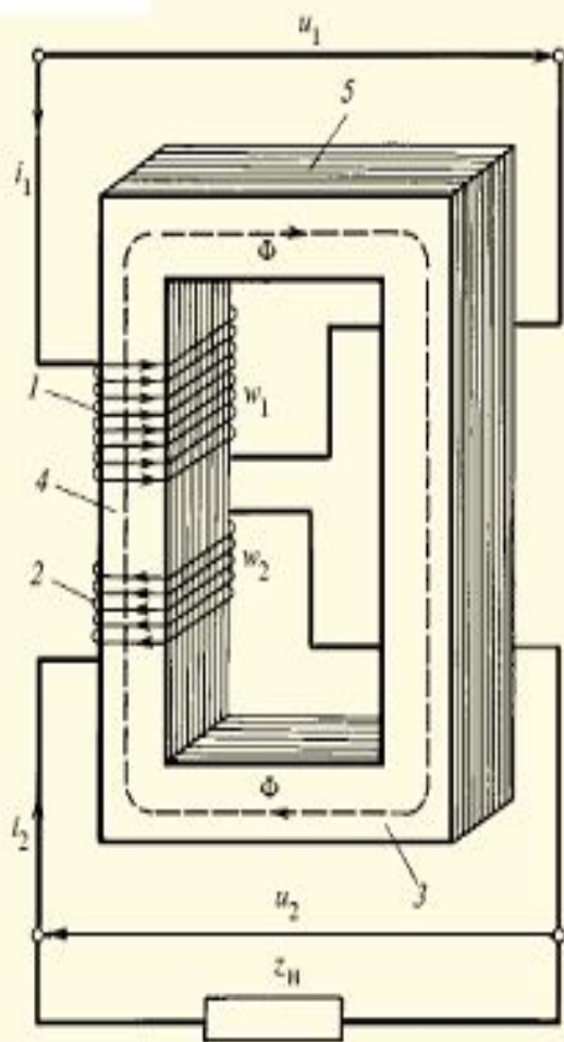
Электромагнитная система однофазного двухобмоточного трансформатора: 1 — первичная обмотка; 2 — вторичная обмотка; 3, 4, 5 — магнитопровод: 4 — стержень магнитопровода; 3, 5 — ярма магнитопровода
