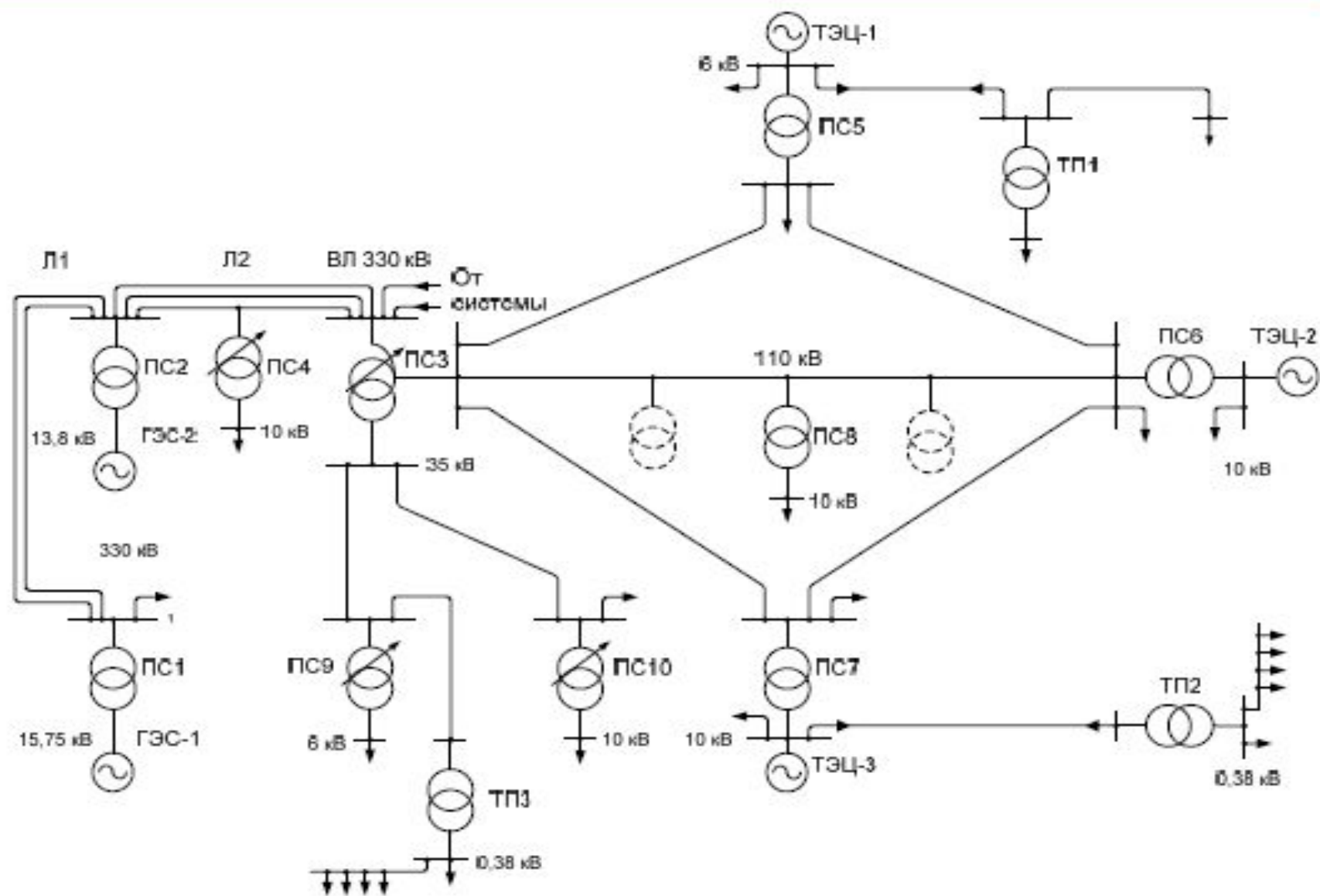
Рис. 1.8. Принципиальная схема передачи и распределения электроэнергии в промышленном районе
