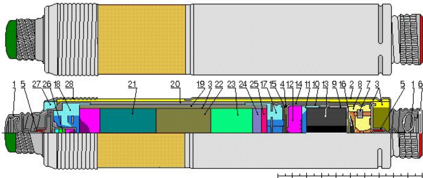
Зажигательно-дымовой патрон ЗДП с ручным броском
