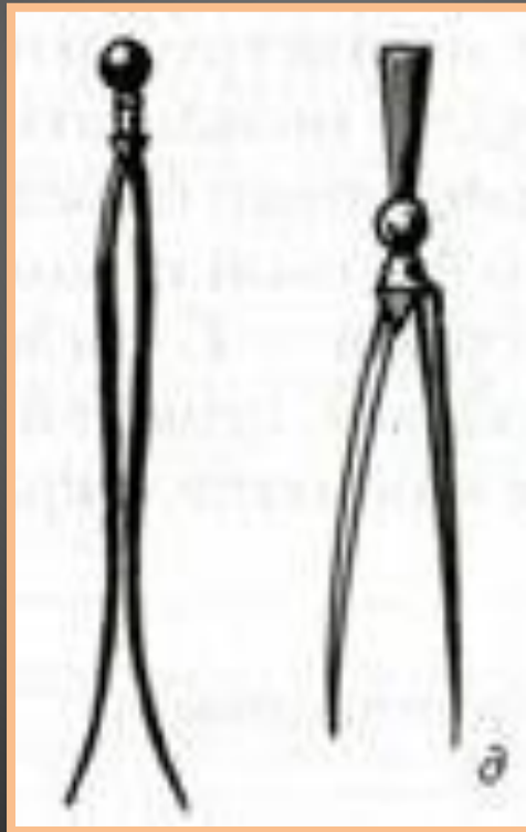
Масштабный циркуль и нутрометр
