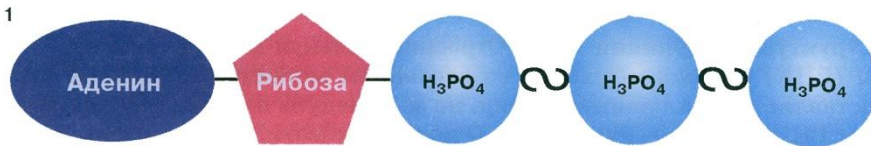
АДЕНОЗИНТРИФОСФОРНАЯ КИСЛОТА
