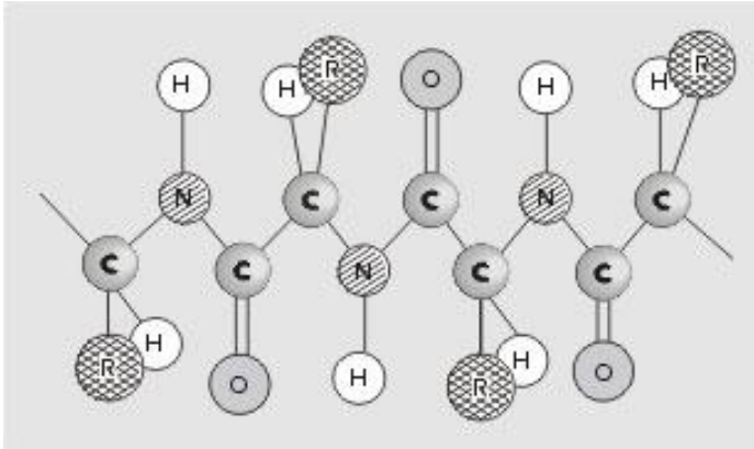
Первичная структура
