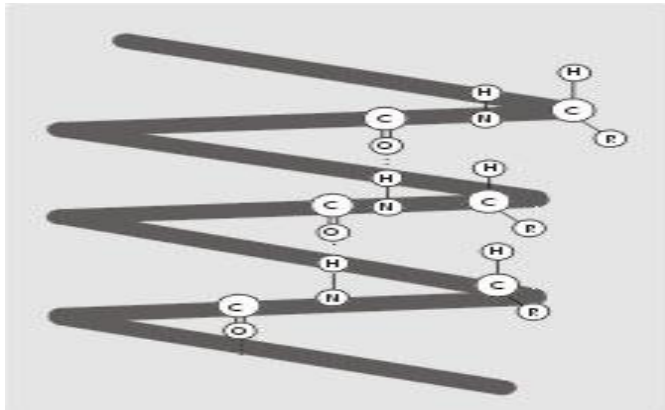
Вторичная структура
