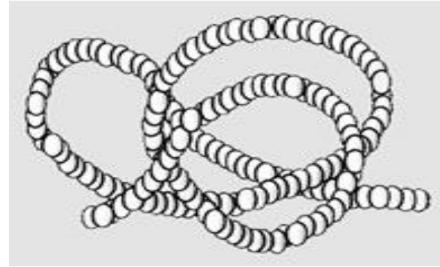
Третичная структура
