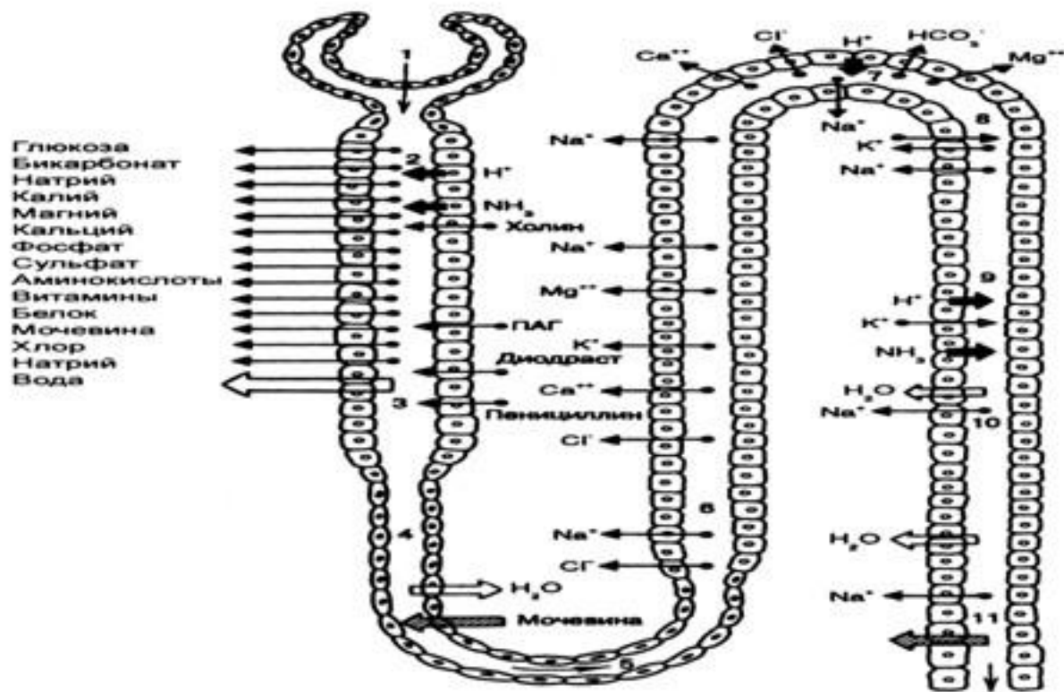
Рис. 3-9. Реабсорбция и секреция электролитов и неэлектролитов в нефроне. 1 — клубочек; 2 — проксимальный извитой каналец; 3 — проксимальный прямой каналец; 4 — тонкое нисходящее колено петли Генле; 5 — изгиб петли Генле; 6 — толстое восходящее колено петли Генле; 7 — дистальный извитой каналец; 8 — связующий отдел; 9 — собирательная трубка наружного мозгового вещества; 10 — собирательная трубка внутреннего мозгового вещества; 11 — беллиниев проток. Стрелка, обращённая из просвета канальца, — реабсорбция вещества, в просвет канальца — секреция [Наточин Ю.В., 2000].
