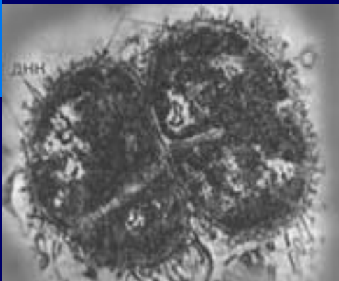
ТЭМ x 50000
