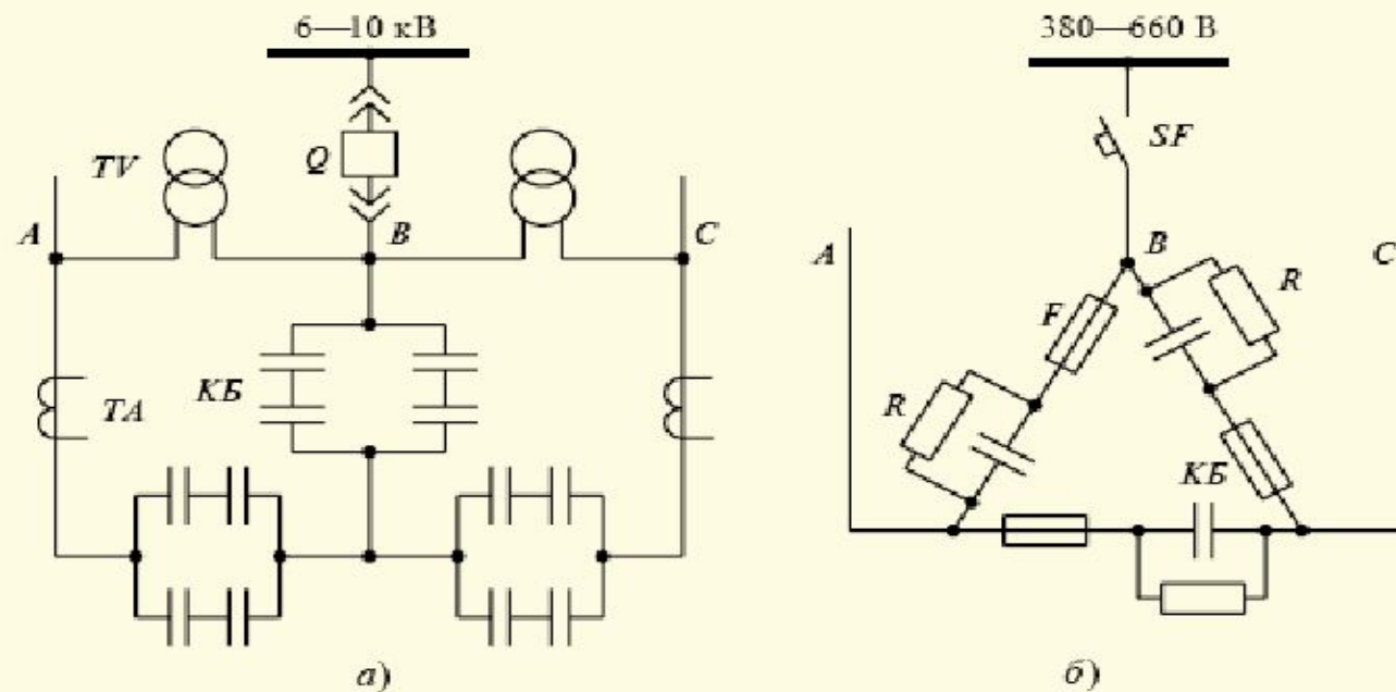
Рис. 8.5. Принципиальная схема одной трехфазной секции КУ: а — для сети 6—10 кВ; б — для сети 380 В
