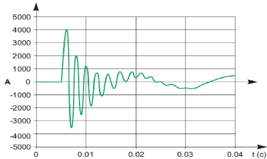
Рис.6. Ток включения
