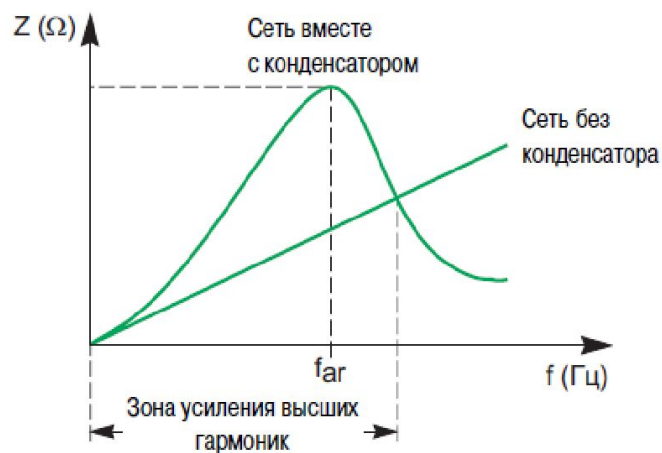
Рис. 14. Модуль сопротивления Z в зависимости от частоты.
