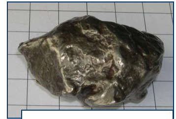
Железо самородное
