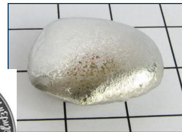
Иридий
