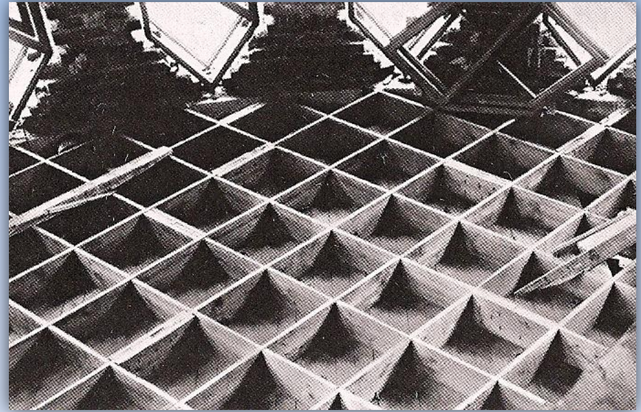
Мембранная конструкция междуэтажного перекрытия, 1927—1929 годы
