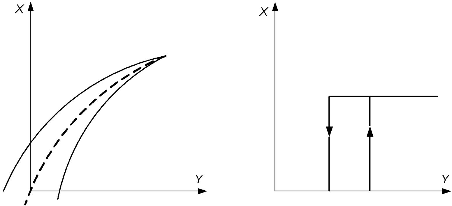
Рис. 1.13. Неоднозначные статические характеристики
