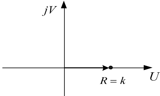
Рис. Амплитудно-фазовая частотная характеристика безынерционного звена
