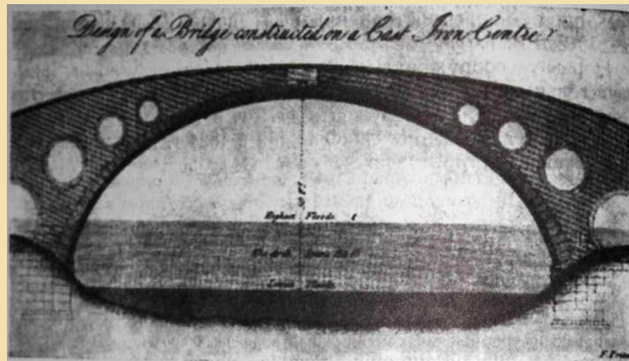
Первый чугунный мост через реку Северн в Колбрук Дейл, 1799 г. Англия
