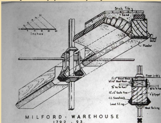
Конструкция огнестойкого перекрытия универмага. Уильям Стратт. 1792—1793 гг.
