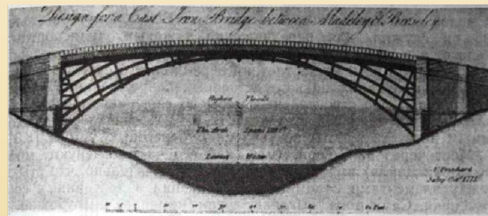
Рис. 20.8. Вариант проекта чугунного моста архитектора Притчарда
