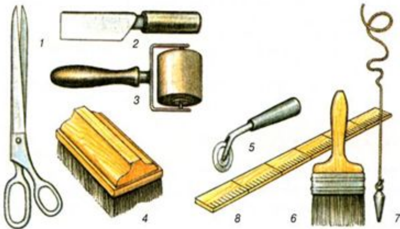
Рис. 186. Инструменты для оклеивания стен обоями: 1 — ножницы; 2 — нож; 3 — валик; 4 — щетка-гладилка; 5 — роликовый нож для обрезки обоев в углах; 6 — кисть для смазывания кромок; 7 — отвес; 8 — линейка с делениями
