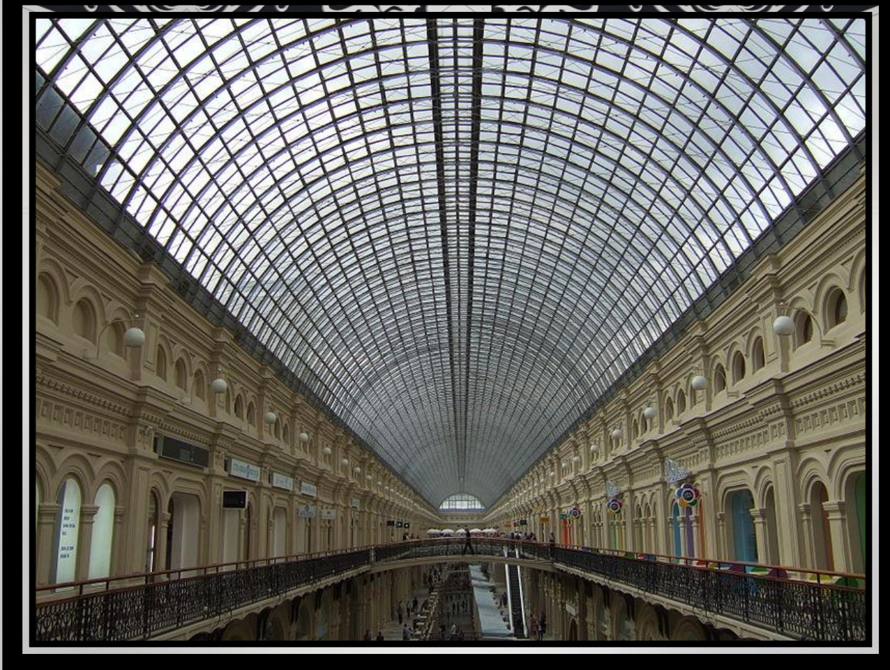
Металло-стеклянные перекрытия ГУМа
