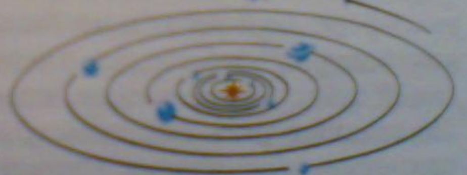
Важнейшие этапы формирования планет.
