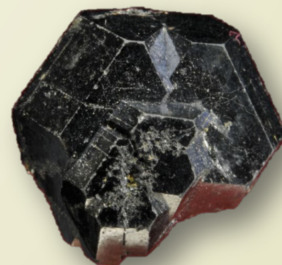
уранинит \text{UO}_2
