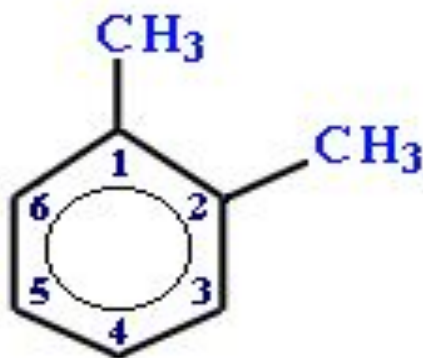
1,2-Диметилбензол
