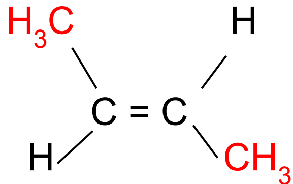
Cis -бутен-2
