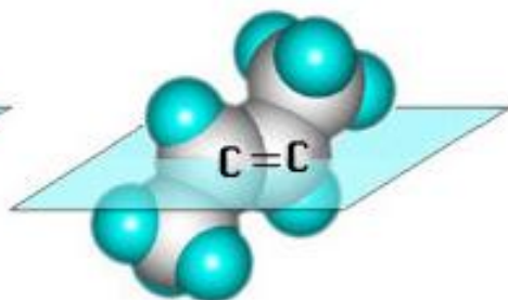
транс-изомер
