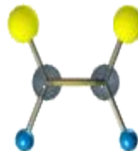
цис-
