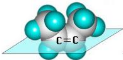
цис-изомер
