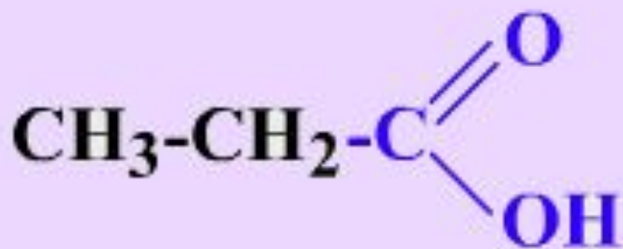
пропановая кислота
