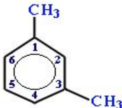
1,3-Диметилбензол
