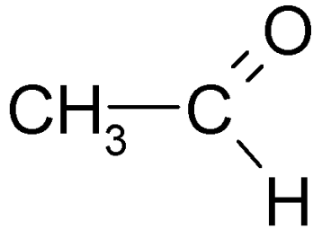
ацетальдегид
