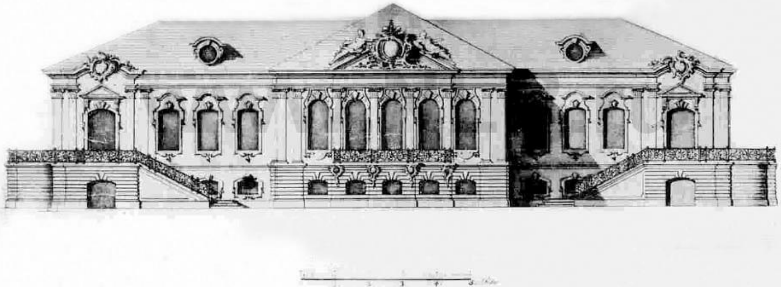
Графъ В. де-Растрелли. Проектъ Среднерогатскаго дворца.
