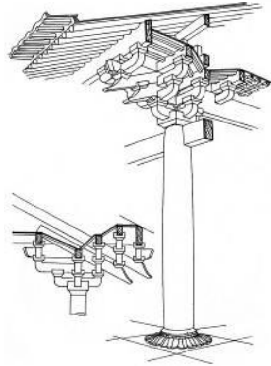
Рис. 1.17. Конструкция доу-гун в кровлях китайских домов
