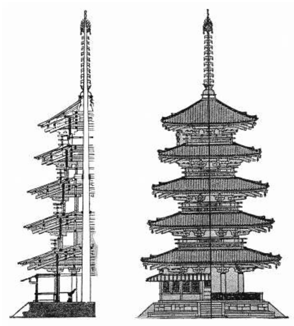
Рис. 10. а – поперечный разрез пагоды.
