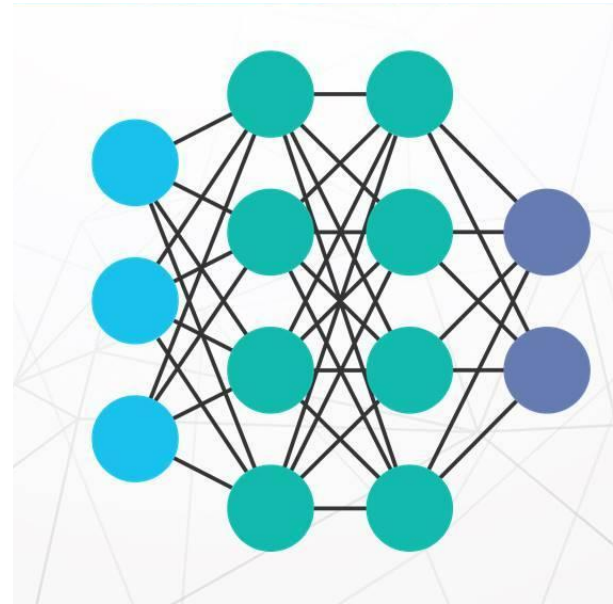
Neuron net
