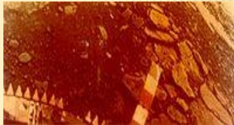
Цветная панорама поверхности Венеры, сделанная советским аппаратом «Венера-13»
