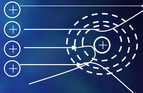
\alpha -частицы
