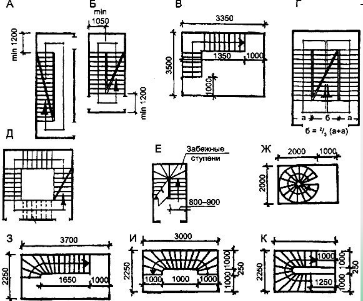
Рис.2. Виды лестниц: А - одномаршевая, Б, В - двухмаршевая, Г, Д - трех- и четырехмаршевые, Е - внутриквартирная с забежными ступенями, Ж - винтовая; З, И, К - круговые, Л - обозначения лестниц на планах
