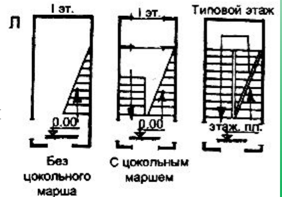
Рис.2. Виды лестниц: А - одномаршевая, Б, В - двухмаршевая, Г, Д - трех- и четырехмаршевые, Е - внутриквартирная с забежными ступенями, Ж - винтовая; З, И, К - круговые, Л - обозначения лестниц на планах
