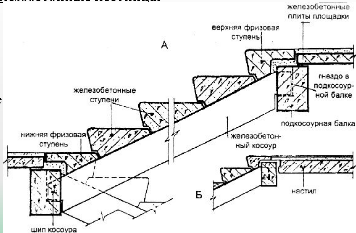
Рис.13. Мелкоэлементная лестница по железобетонным косоурам
