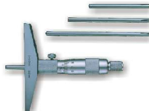
● ГЛУБИНОМЕРЫ МИКРОМЕТРИЧЕСКИЕ
