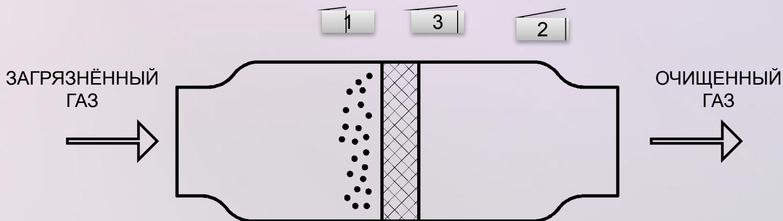
РИСУНОК 1. СХЕМА ЭЛЕКТРОФИЛЬТРА
