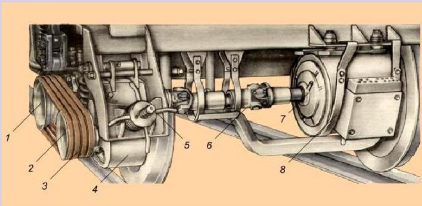
Рис.1. Расположение текстропно-редукторно-карданного привода: 1 — ведущий шкив; 2 — ведомый шкив, 3 — четыре приводных ремня; 4 — редуктор; 5 — натяжное устройство; 6 — карданный вал; 7 — генератор; 8 — предохранительное устройство
