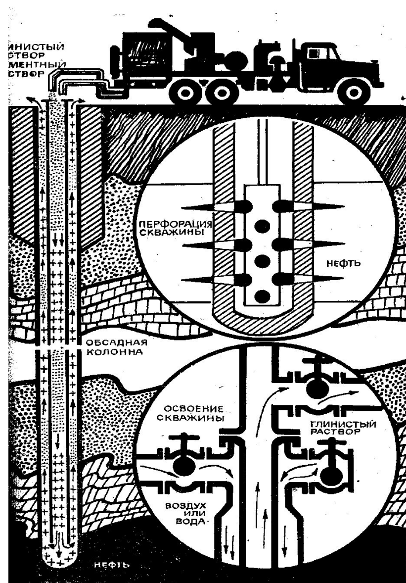
Принцип бурения скважин
