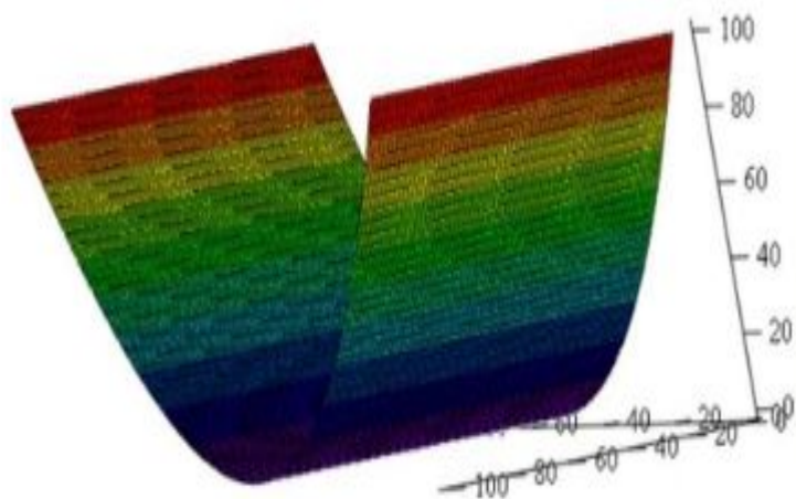
Параболический цилиндр
