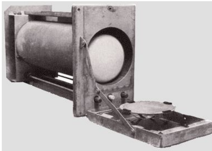
Запоминающая электронно-лучевая трубка Фредерика Уильямса
