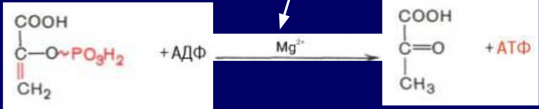
L'ACIDE PYRUVIQUE
