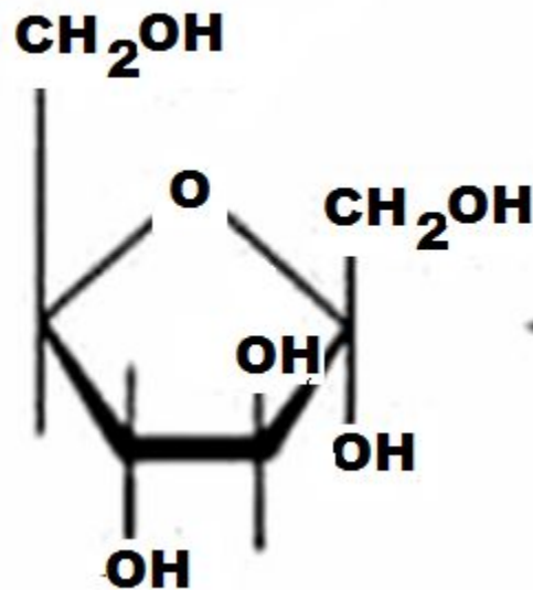
LE FRUCTOSE
