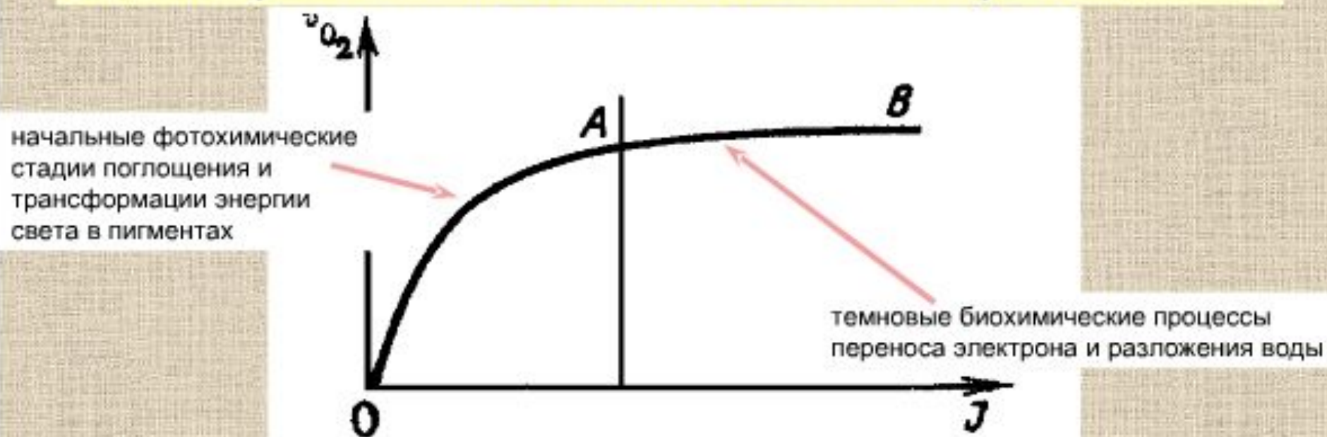
Рис. 1.6. Зависимость скорости выделения кислорода ( v_{O_2} ) от интенсивности освещения ( I ) при фотосинтезе
