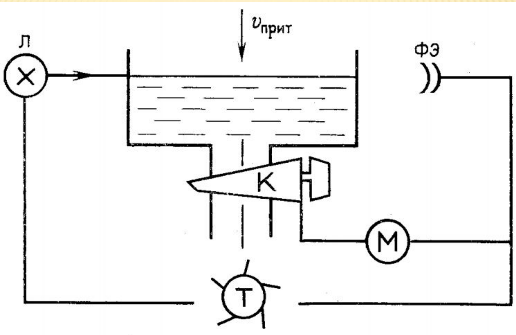
Гидродинамическая модель системы с обратной связью Л – лампа, ФЭ – фотозлемент, К – кран, М – электромотор, Т – турбина
