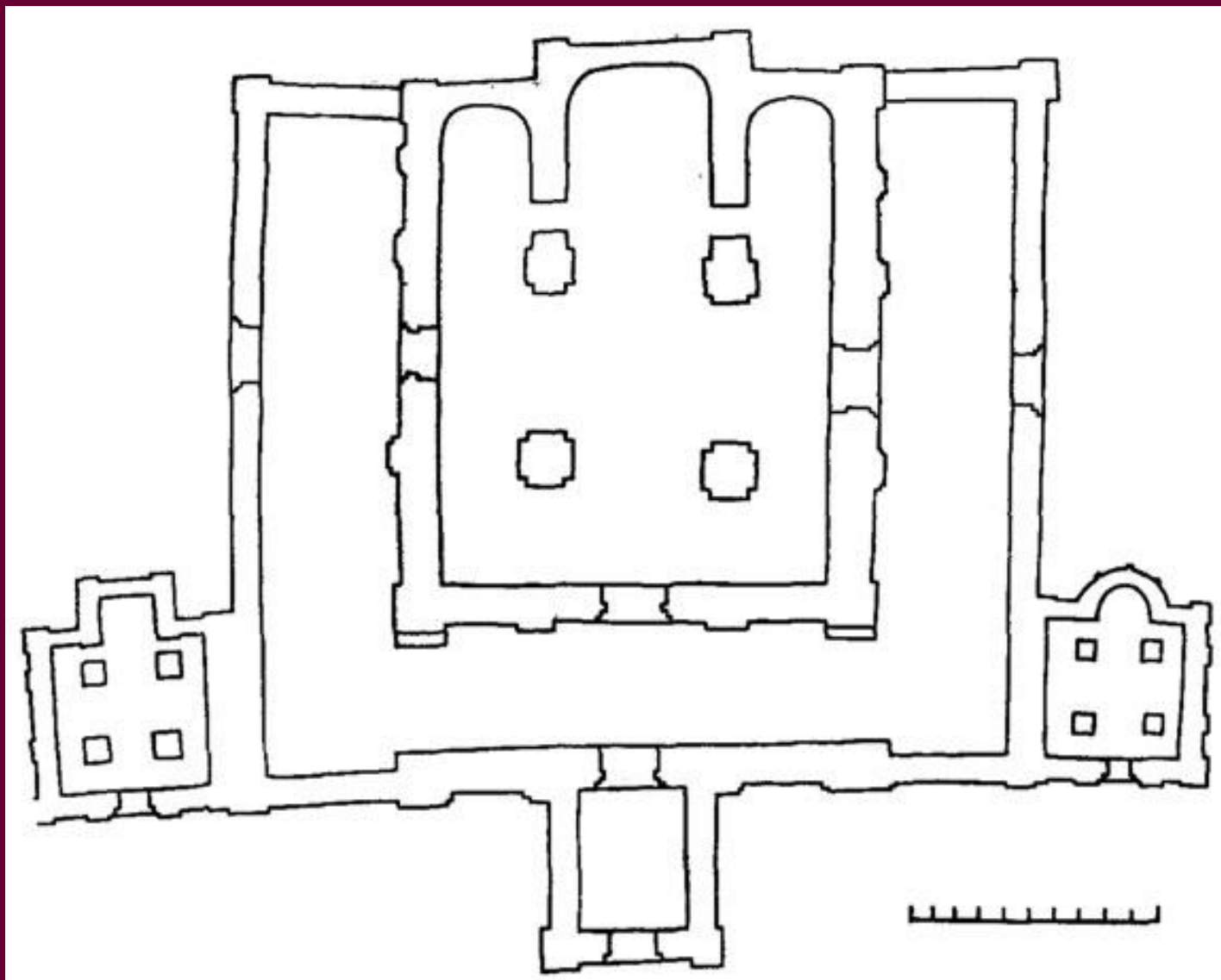
Собор на Протоке. Смоленск. Первая четверть XIII в. План
