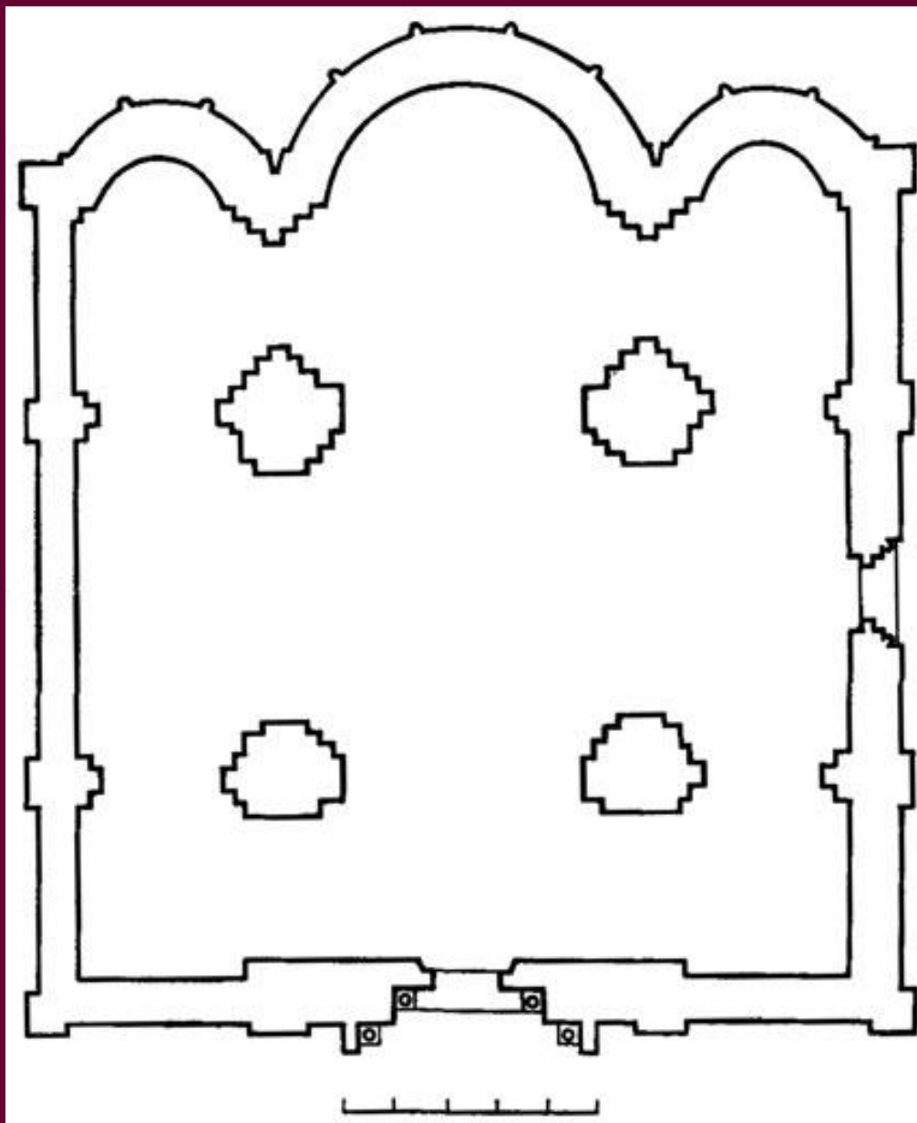
ц. Пантелеймона. Галич. XII – XIII в. План.
