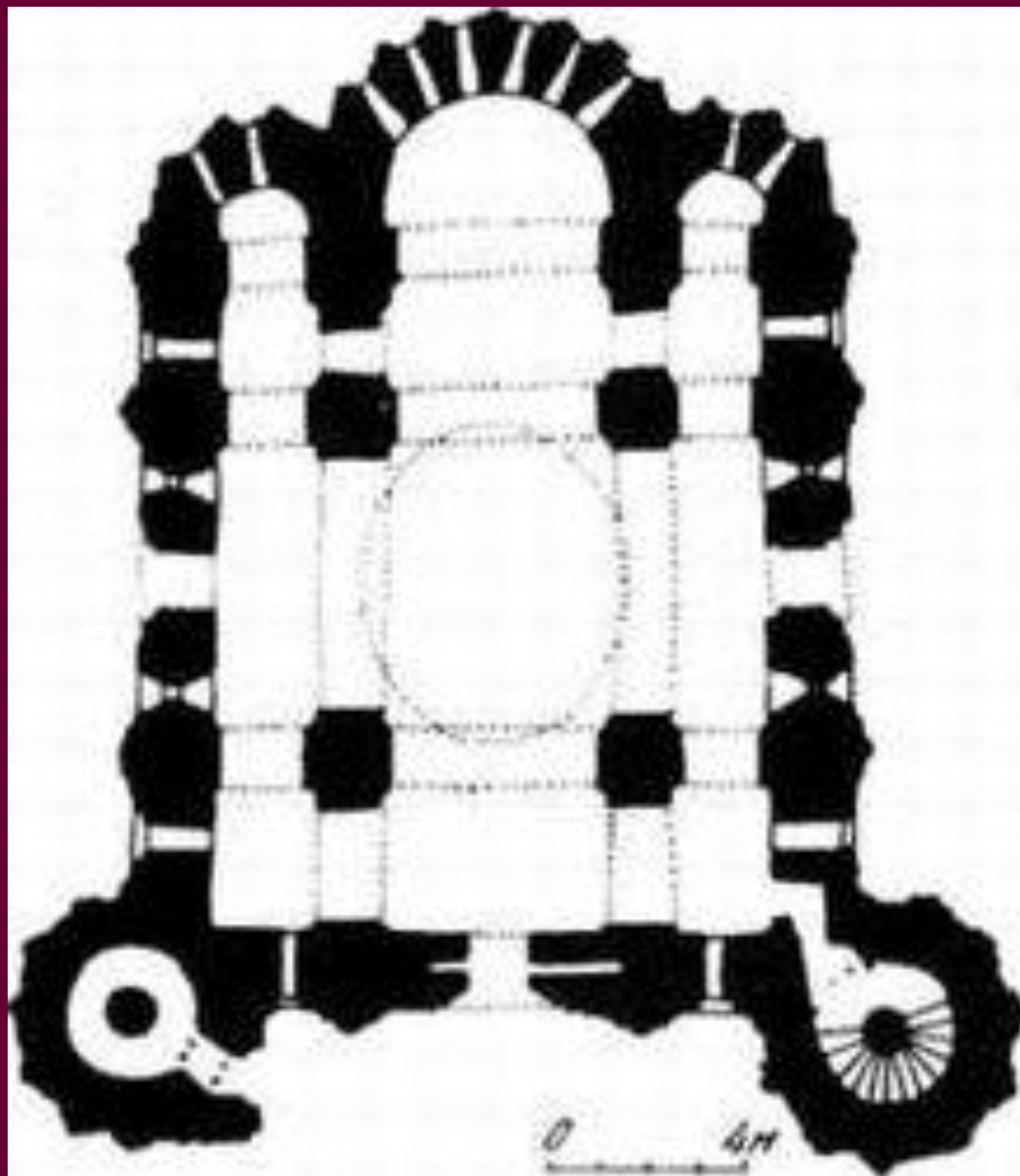
ц. Василя. Овруч. Конец XII в. План
