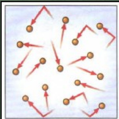
Хаотическое движение молекул газа
