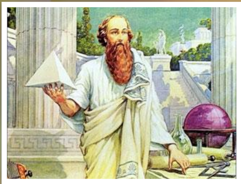
Пифагор
