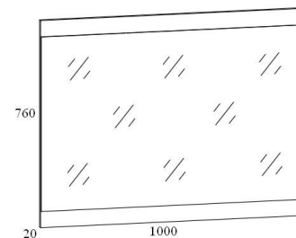
Зеркало S122-LUS/8/10
