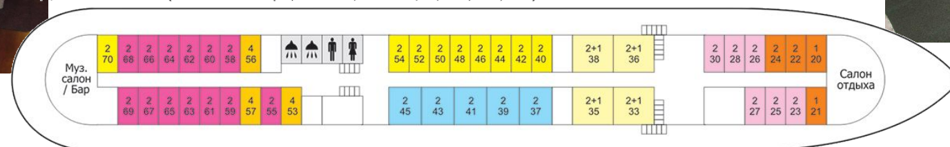
ГЛАВНАЯ ПАЛУБА (Классы Гамма эконом, 2А, 2Б)
