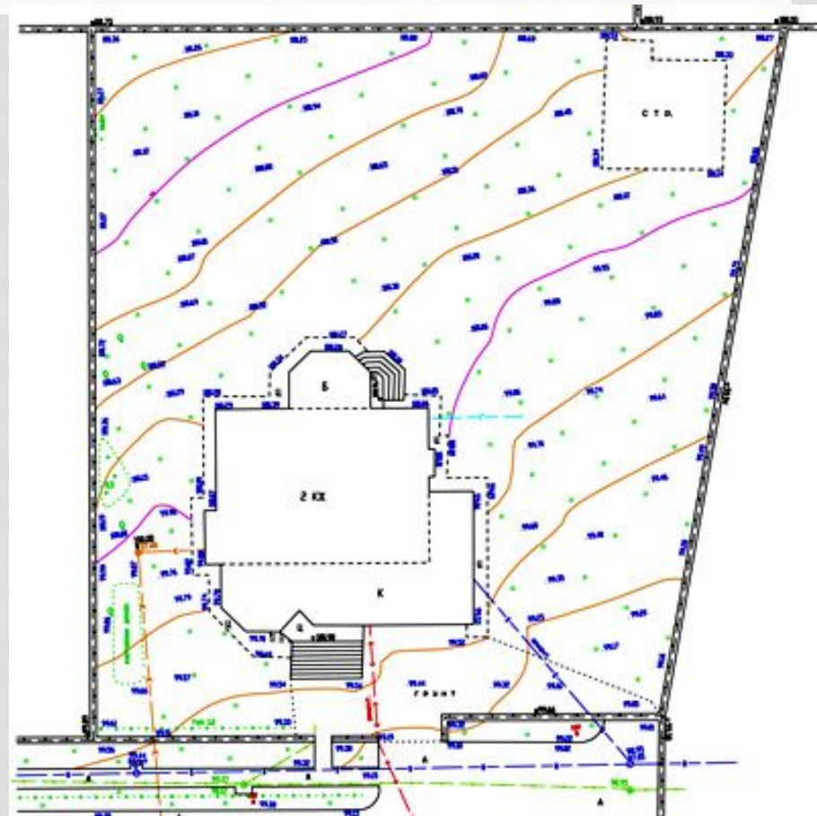
Садовый дворик. Обмерочный чертёж
