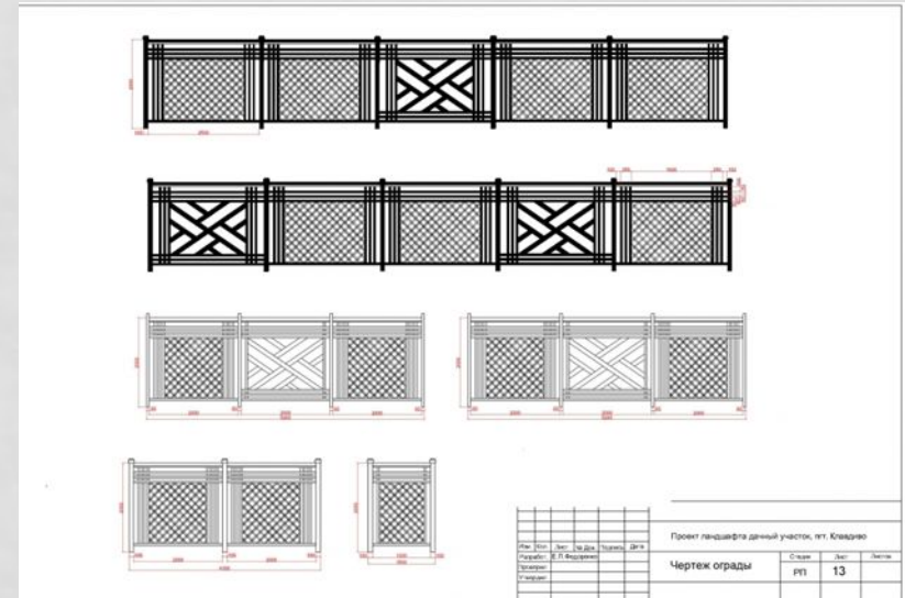
Чертёж ограды
