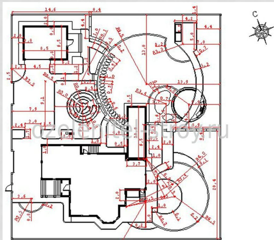
Разбивочный чертёж
