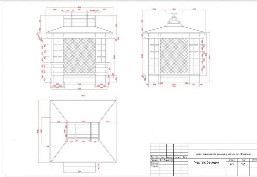
Чертёж беседки
