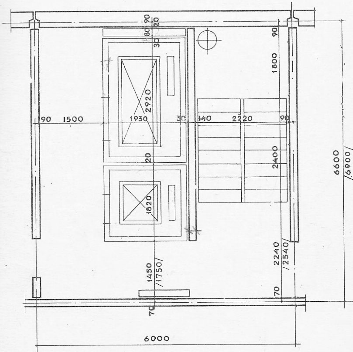
ЛЕСТНИЧНО-ЛИФТОВОЙ УЗЕЛ ЛЛУ7-1 ПЛАН ТИПОВОГО ЭТАЖА
