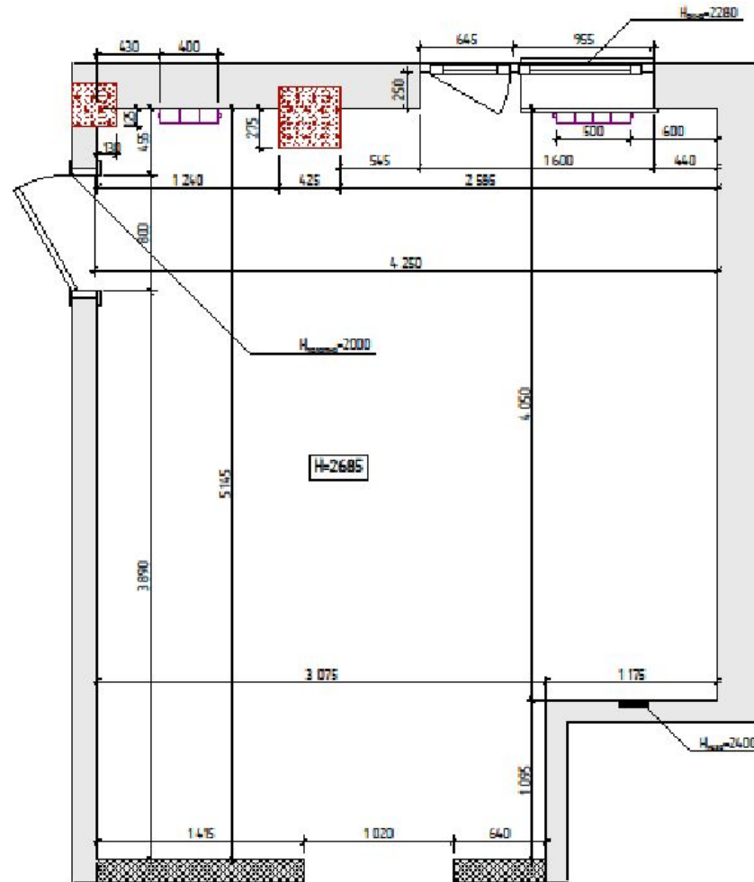
План обмеров
