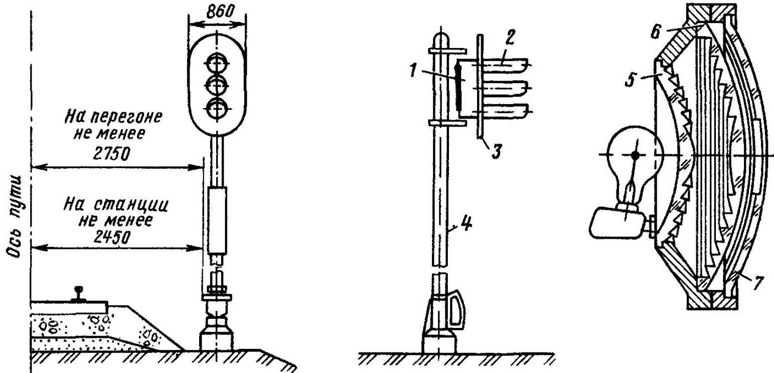
Рис 20.3 Устройство линзового светофора:
