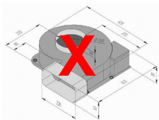
ESL 850.0 Цокольный вентилятор
