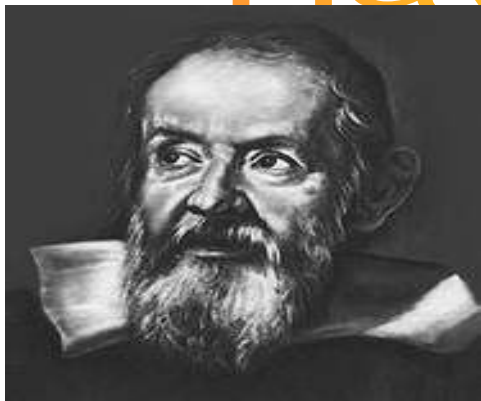
Галилео Галилей
