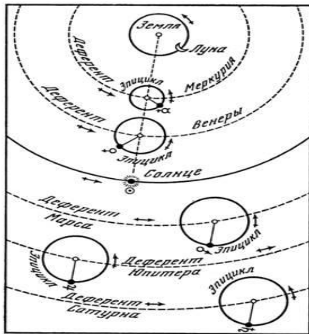
Рис. 24. Система мира Птолемея
