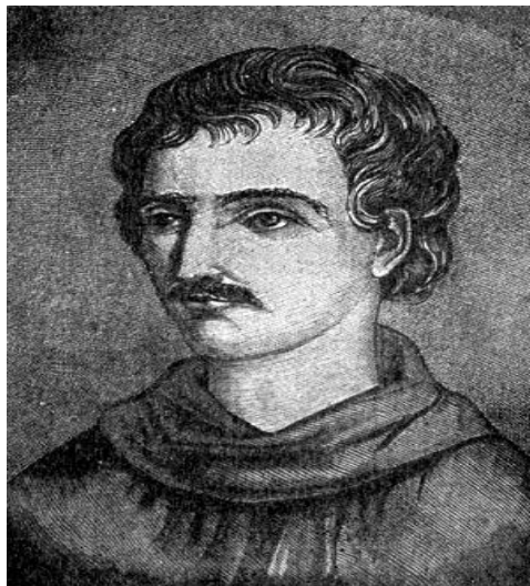
Джордано Бруно
