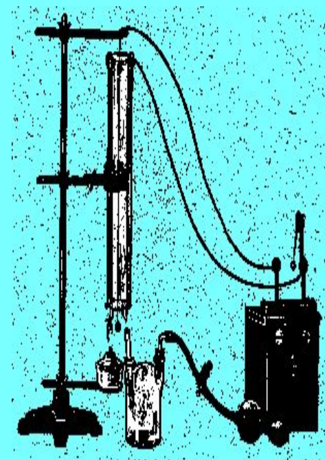
Рис. 12.5. Электрофилтр
