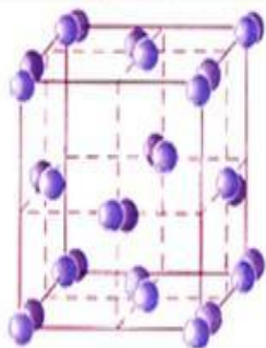
Кристаллические решетки алмаза (слева) и графита (справа)
