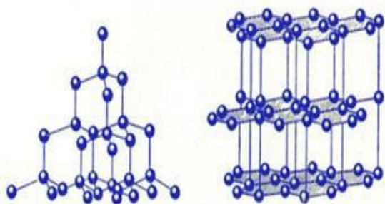
Кристаллические решетки алмаза (слева) и графита (справа)
