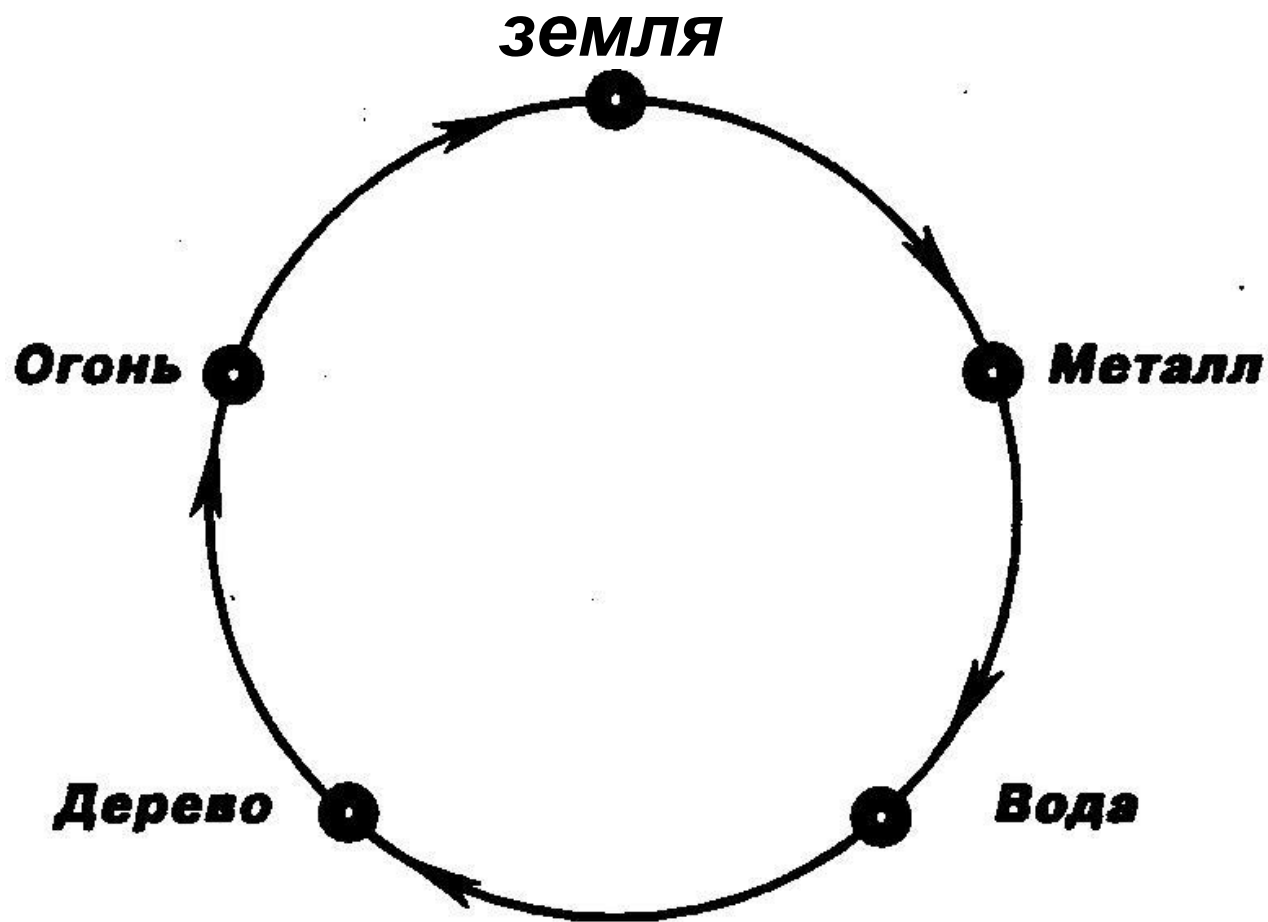
Рис. 4. Закон созидания.
