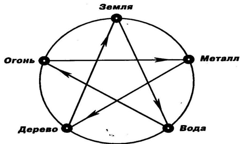
Рис. 5. Закон угнетения
