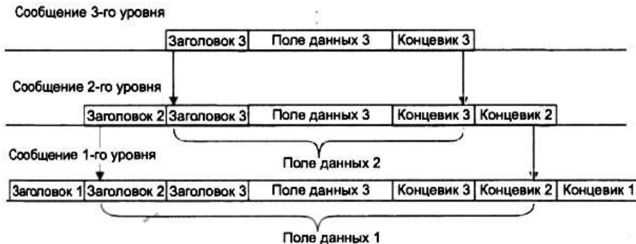
Рис. 2. Вложенность сообщений различных уровней
