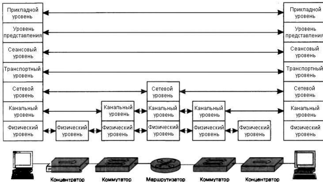
Рис. 1. Соответствие функций различных устройств сети уровням модели OSI
