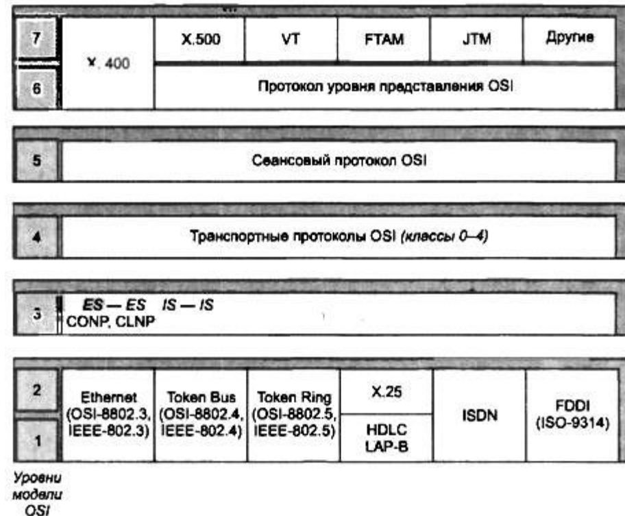
Рис. 1. Стек протоколов OSI
