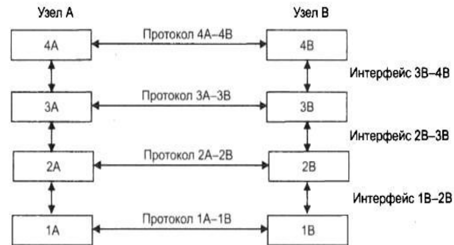
Рис. 1 Взаимодействие двух узлов
