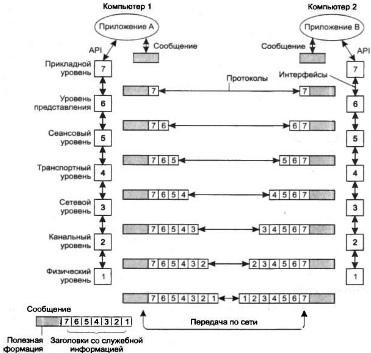
Рис. 1. Модель взаимодействия открытых систем ISO/OSI
