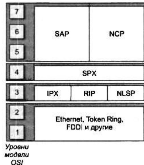
Рис. 1. Стек протоколов IPX/SPX
