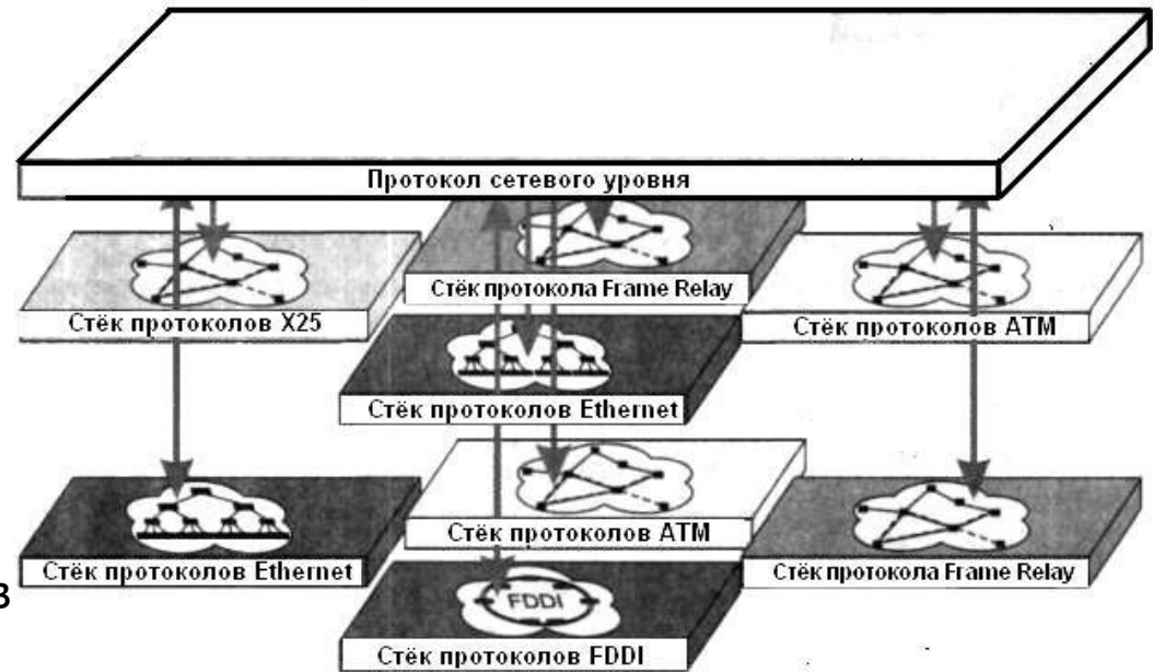
Рис. 1. Необходимость сетевого уровня
