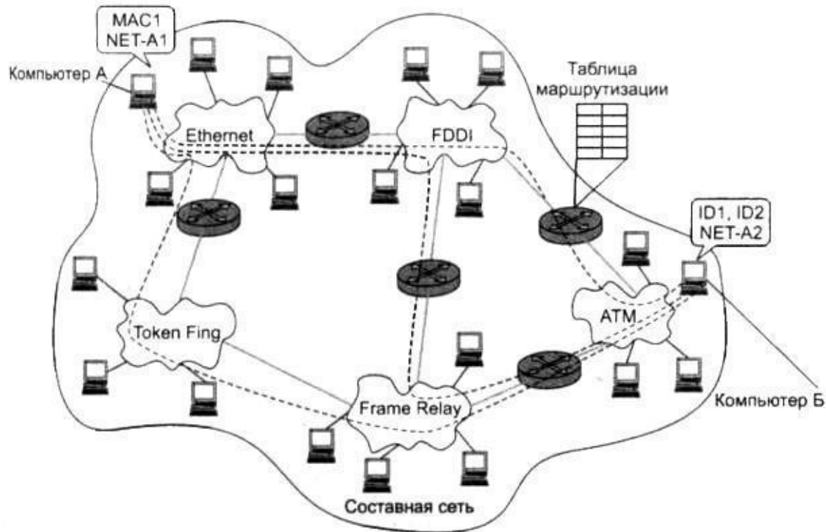
Рис.2. Пример составной сети
