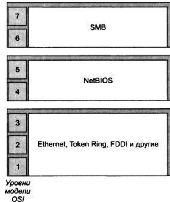
Рис. 1. Стек NetBIOS/SMB
