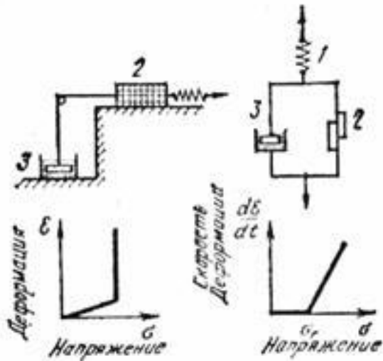
Рис. 1.22. Модель Шведова - Бингама
