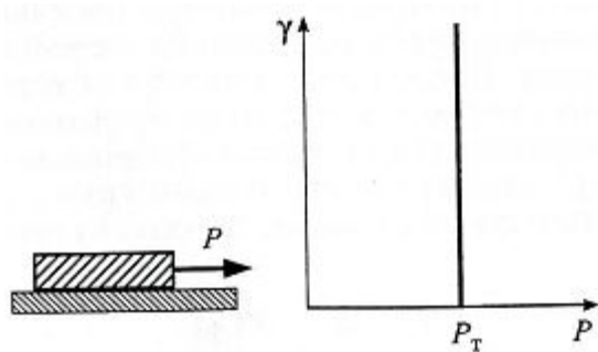
Модель идеально пластического тела Сен-Венана—Кулона
