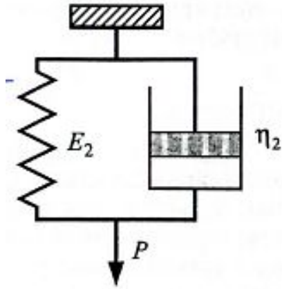
Рис. VI.18. Модель Кельвина—Фойгта
