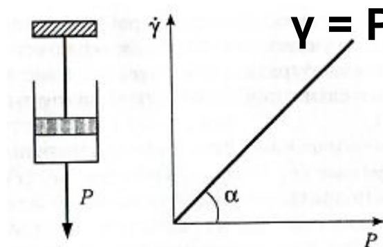
Модель идеально вязкого тела Ньютона
