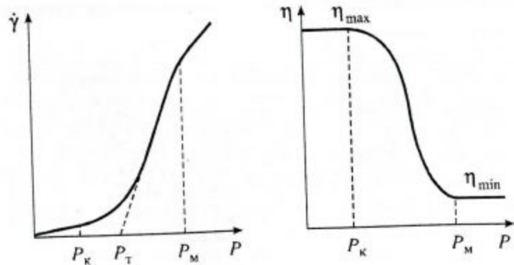
Рис. VI.6. Реологические кривые течения и эффективной вязкости дисперсных систем с коагуляционно-тиксотропными структурами
