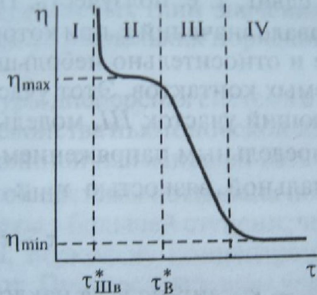
Рис. IX-21. Полная реологическая кривая в координатах \eta - \tau
