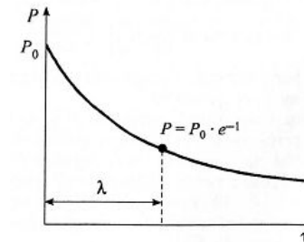
Кривая релаксации напряжения
