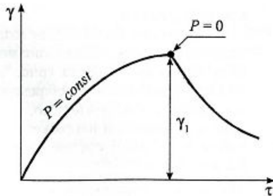
Деформационная кривая модели Кельвина—Фойгта
